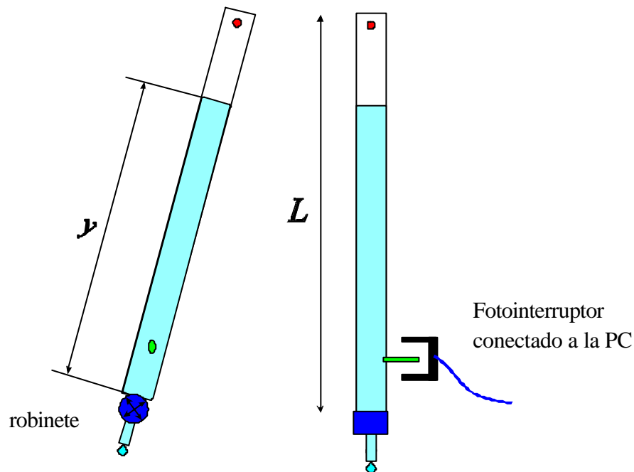
Figura 1: Esquema de un péndulo goteador.
