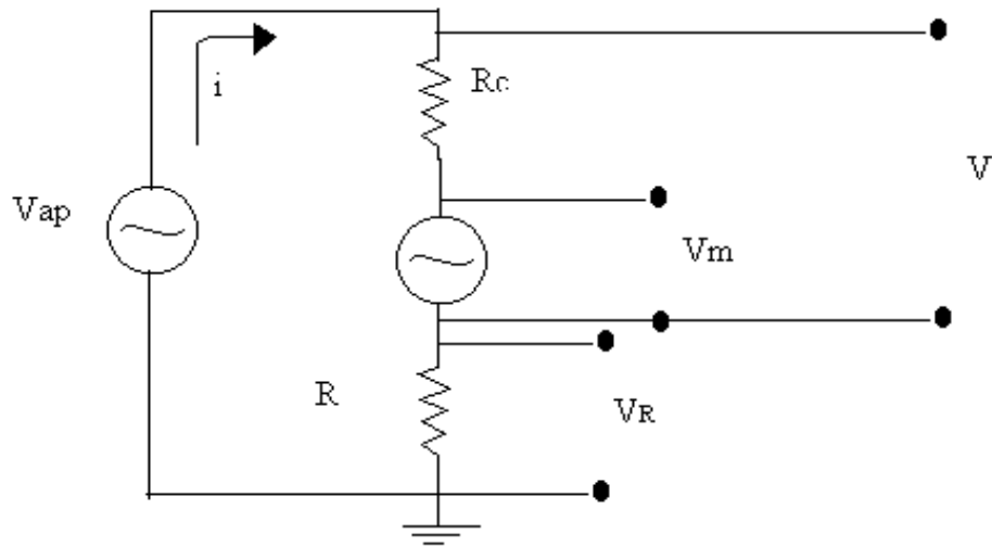
Figura 1 Circuito modelo. R_c = 2.03 \text{ K}\Omega R = 9.83 \text{ K}\Omega . No se tiene en cuenta a la resistencia interna. V_m es proporcional a la velocidad de la aguja ( d\theta/dt ). V_r es proporcional a la fuerza restauradora F_{ap} , la cual a su vez es proporcional a la corriente. V_m = V - i R_c V_R = iR
