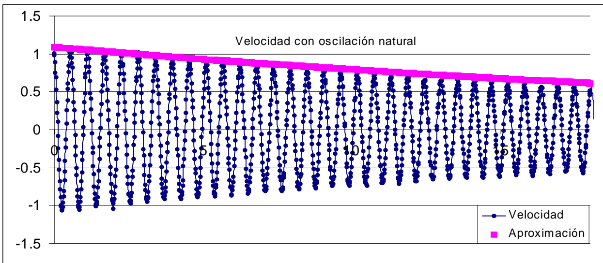
Figura 3 Velocidad en función del tiempo para oscilación natural. La constante de amortiguación \gamma = 0.029 \pm 0.003 . La frecuencia natural determinada con la herramienta FFT es f_o = 1.78 \pm 0.05 Hz
