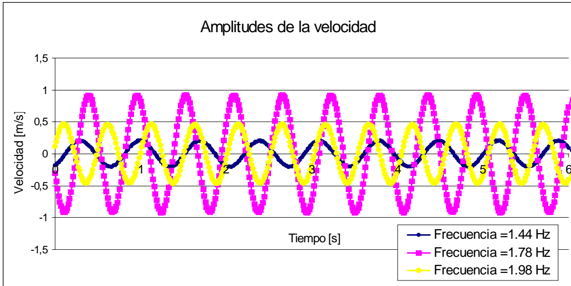
Figura 4 Amplitud de la velocidad para distintas frecuencias excitadoras.
