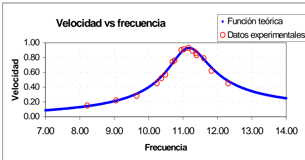
Figura 5 Variación de la amplitud de la velocidad con la frecuencia. La frecuencia natural (igual a 2 \pi f_0 ) es igual a 11.2 \pm 0.2 Hz. \gamma = 0.030 \pm 0.002
