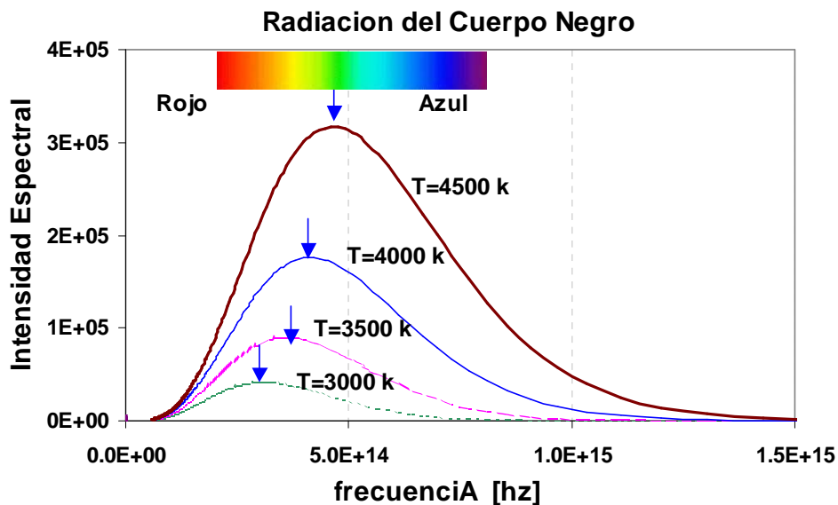
Figura A.3. Espectro de la radiación electromagnética de un cuerpo negro a distintas temperaturas, representadas por la letra T . Las flechas indican la posición del máximo de radiación a cada temperatura. En la parte superior se ilustran los colores de la luz, correspondiente a las frecuencias visibles, indicadas en el eje horizontal.
